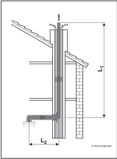
Odprowadzenie spalin w szachcie typu C 93
