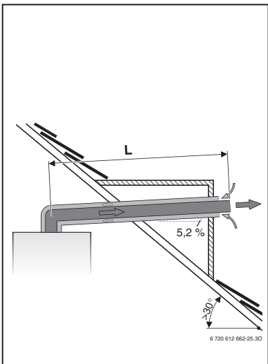
Odprowadzenie spalin w szachcie typu C 13
