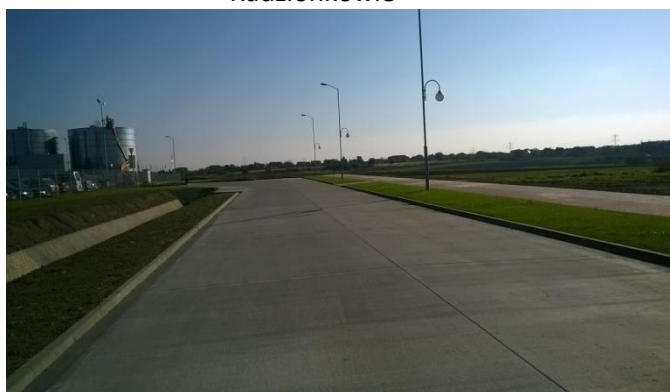
Budowa drogi zbiorczej o nawierzchni betonowej szerokości 7,0 m na odcinku od km 0+23,2 do 0+380,0 km
