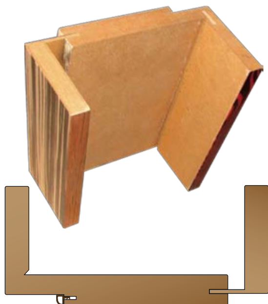
Przekrój ościeżnicy
