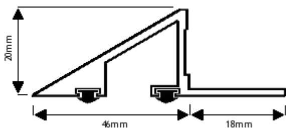
RAMA NAJAZDOWA
