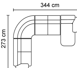
008 SECT.(16+29+28+49)
