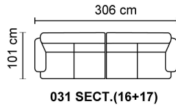
031 SECT.(16+17)
